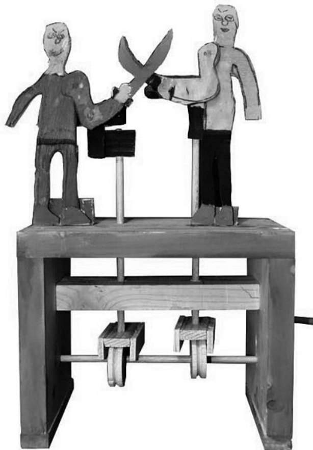
Getriebe 1. Klasse
